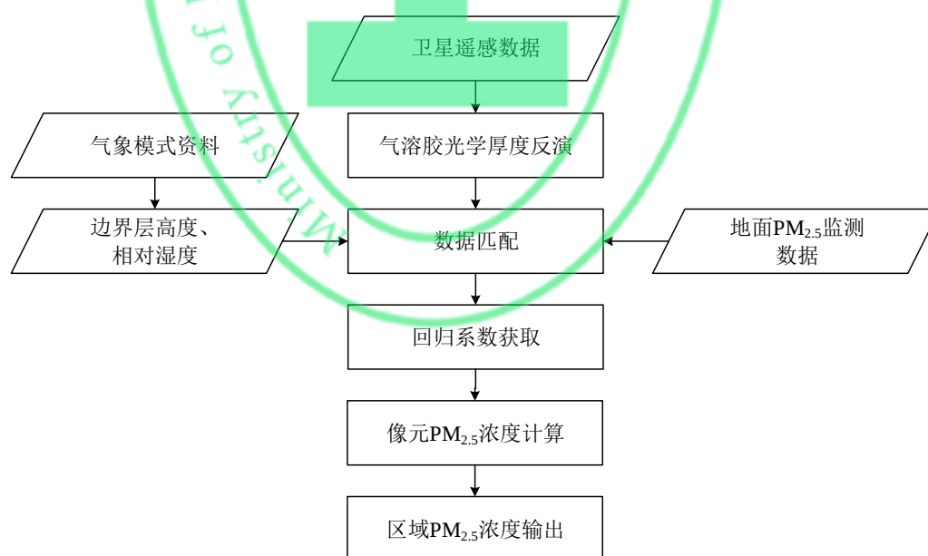
图 1 陆地区域 \text{PM}_{2.5} 质量浓度卫星遥感监测流程图
